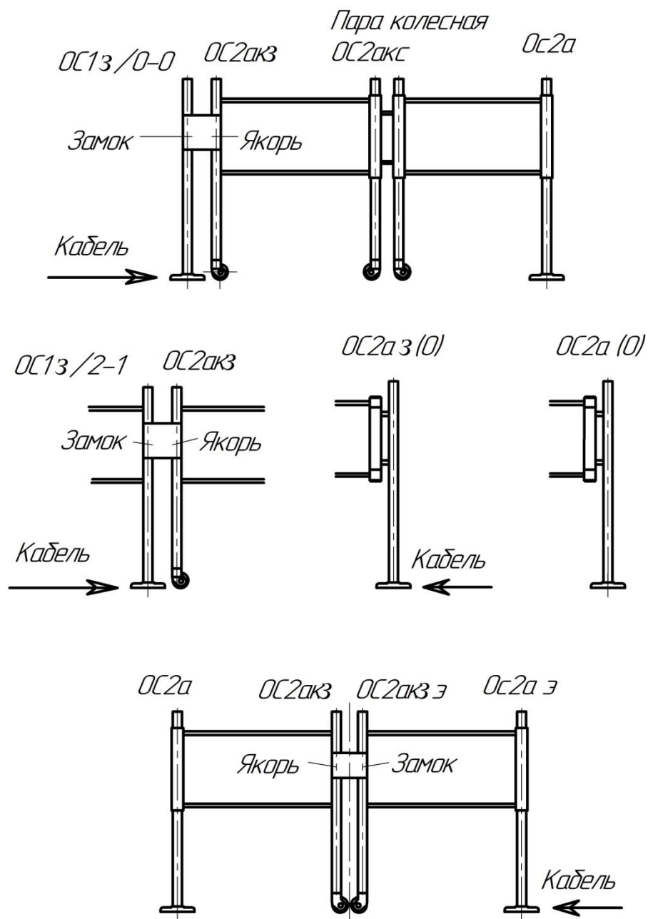
Рис. 9. Виды стоек ограждений с электромагнитным замком
