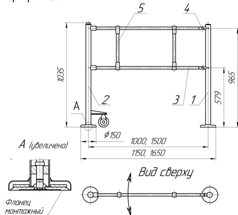
Рис.10.Конструкция, габаритные размеры и комплектация ограждения ОС2акп
